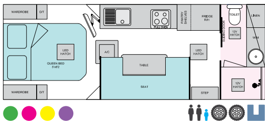
V5-3 20'6"
