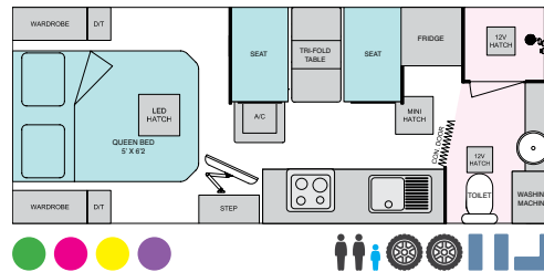
V2-1 19'
